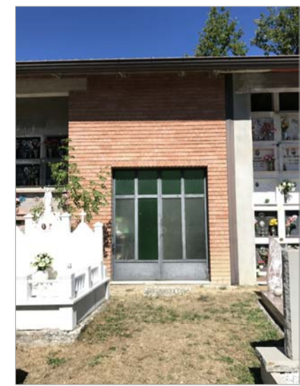
Realizzazione di intonaco su muratura della cappella e rifacimento portoncino
