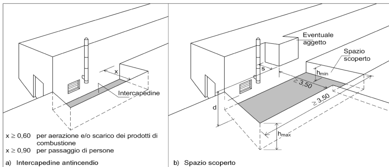
Figura 81.6 Intercapedine antincendio e spazio scoperto secondo il D.M. 30 novembre 1983
